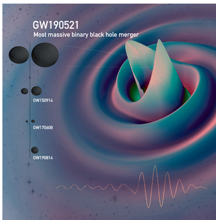
Рис. 1. Цифровая модель процесса слияния двух наиболее массивных чёрных дыр, соответствующая наблюдению GW190521 от 21 мая 2019 г. [7]
