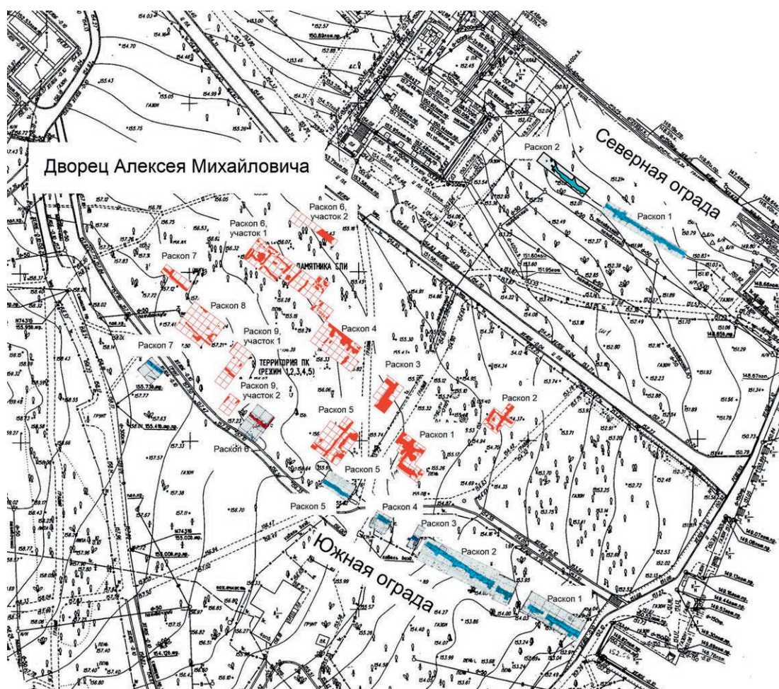
Ил. 10. Раскопы 2005 г. на геодезической подоснове участка дворца. Сводный план. Синим показаны раскрытые участки кирпичной ограды, красным — опорные кладки, фундаменты печей и стенки сооружений в составе дворца
