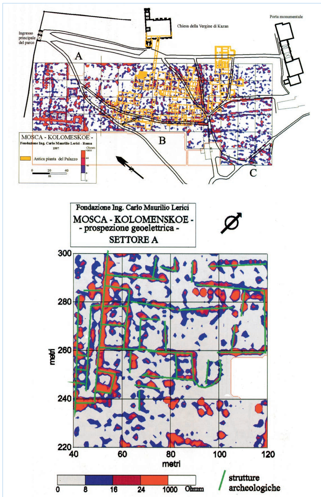
Ил. 13. Дворец в Коломенском: схема плана на основании архивных чертежей (жёлтым) и наложенные на него линии фундаментов согласно геофизическому зондированию участка 1997 г. (по: Zolese P., Nalesini O., Cucarzi M., 1999. S. 38, 39)
