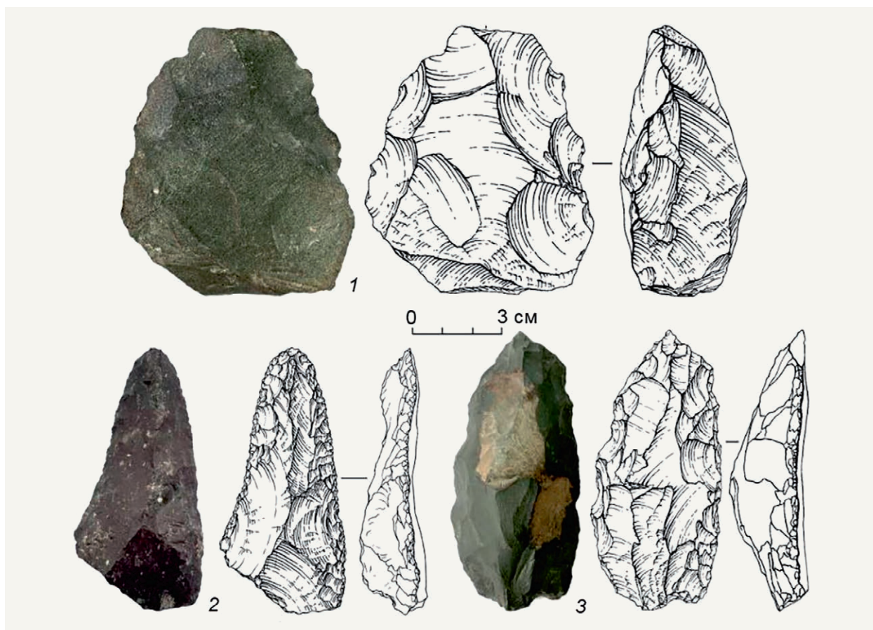
Рис. 2. Древнейшие каменные орудия денисовцев: 1 — вентрально-утончённый скол; 2, 3 — скребла
