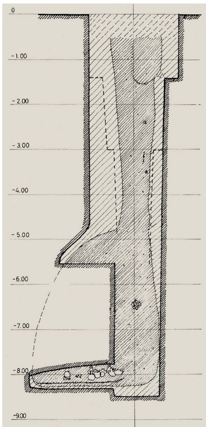
Рис. 4. Конструкция «шахтной гробницы», культура Викас (Перу)
