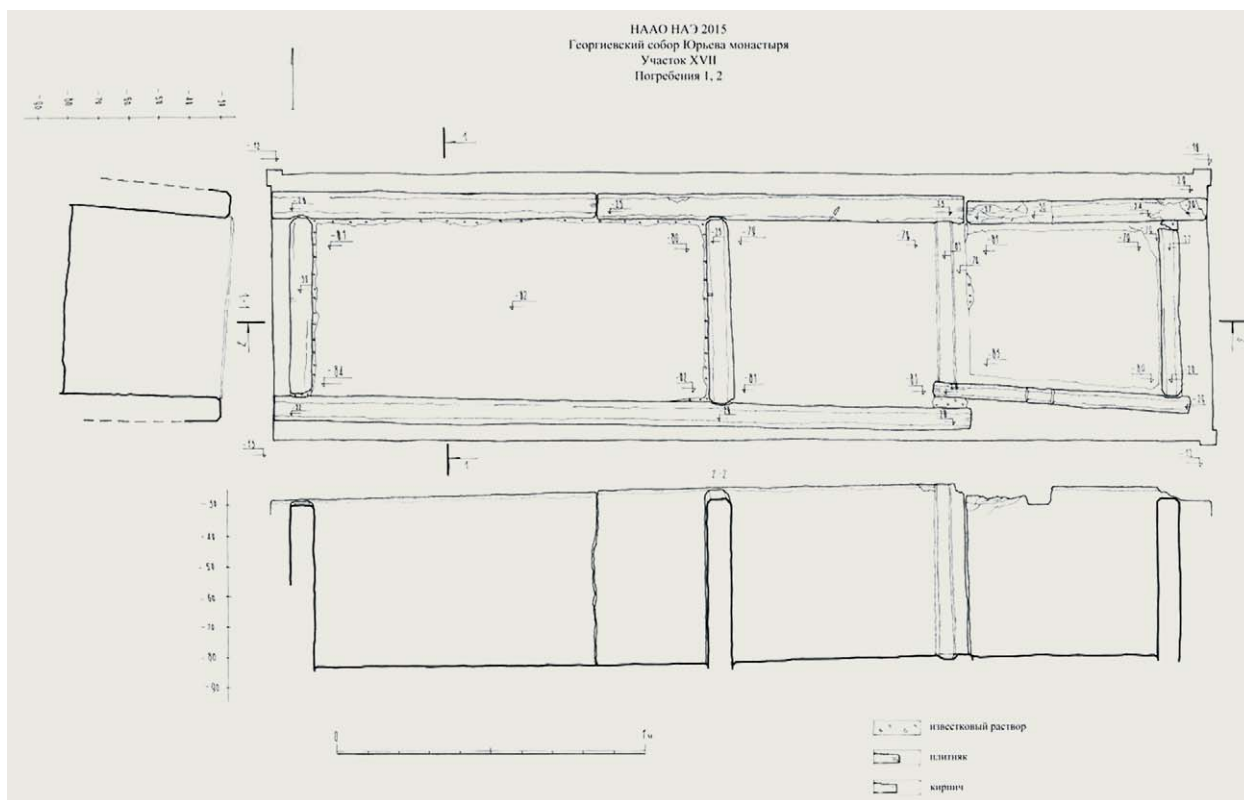
Ил. 7. Саркофаг погребения 1 и 2 (погребения княжичей Изяслава и Ростислава). План и разрезы
