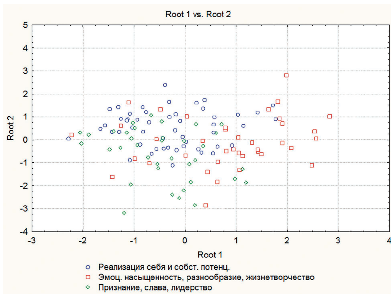
Рис. 4. Диаграмма локализации кластеров на основе дискриминантных функций
