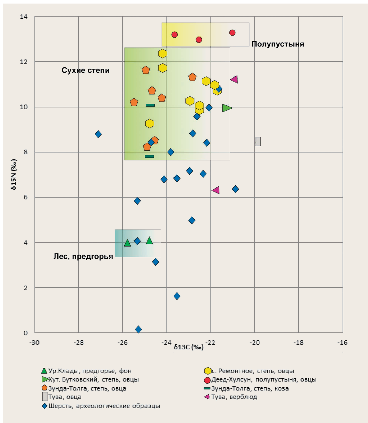
Рис. 6. Изотопный состав азота и углерода кератина археологического шерстяного волокна бронзового века ( \delta^{13}\text{C} ; \delta^{15}\text{N} ) и шерсти современных овец
