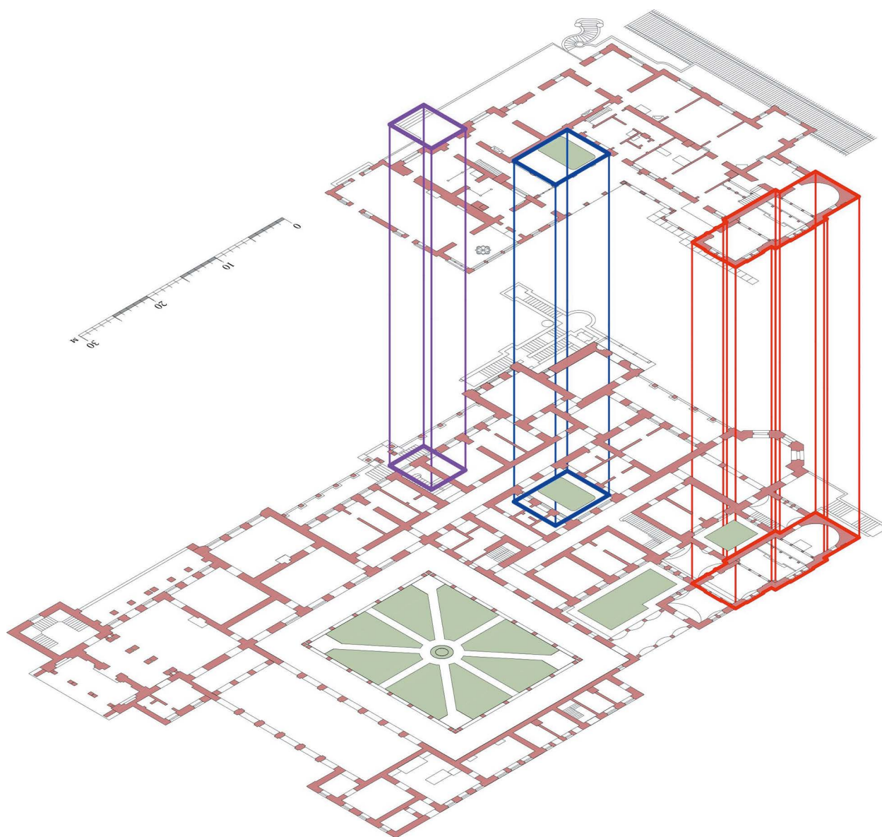
Ил. 2. И.Н. Слюнькова, О.А. Спиридонова. Графическая сравнительная таблица планов старого и нового императорского дворца в Ливадии. 2019. Публикуется впервые
