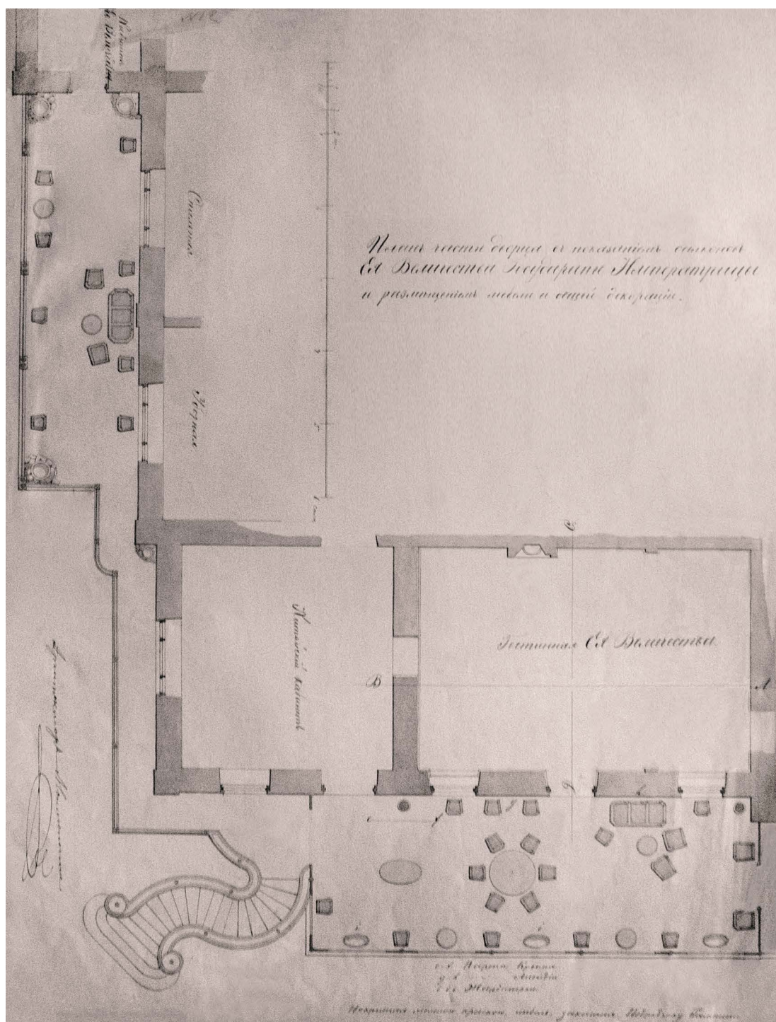
Ил. 5. И.А. Монигетти. Ливадийский дворец. Эскиз фрагмента плана. 1863. НИМ РАХ. Публикуется впервые
