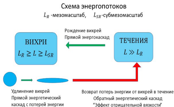
Рис. 2. Схема обмена энергией между течением и вихрем при вытягивании вихря.
