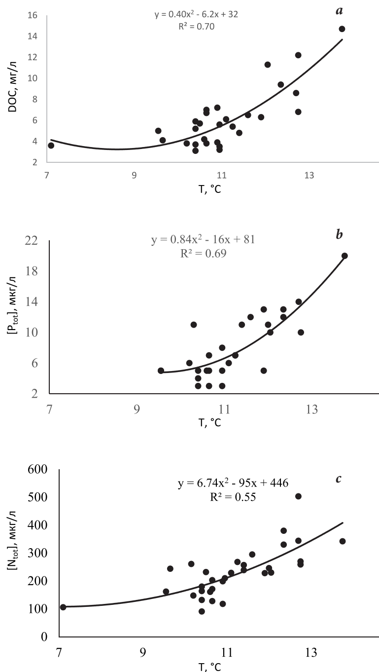
Рис. 4. Зависимости между содержанием растворенного органического вещества DOC в пересчете на углерод (a), общего фосфора ( P_{tot} ) (b), общего азота ( N_{tot} ) (c) и средней температурой приземного слоя воздуха за период 1990–2018 гг.
