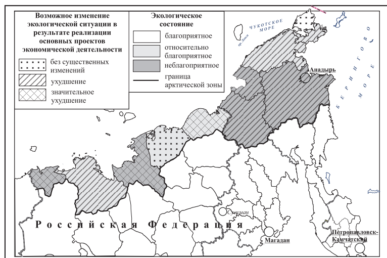
Рис. 3. Экологическое состояние административных субъектов на северо-востоке России и прогноз его возможного изменения.
