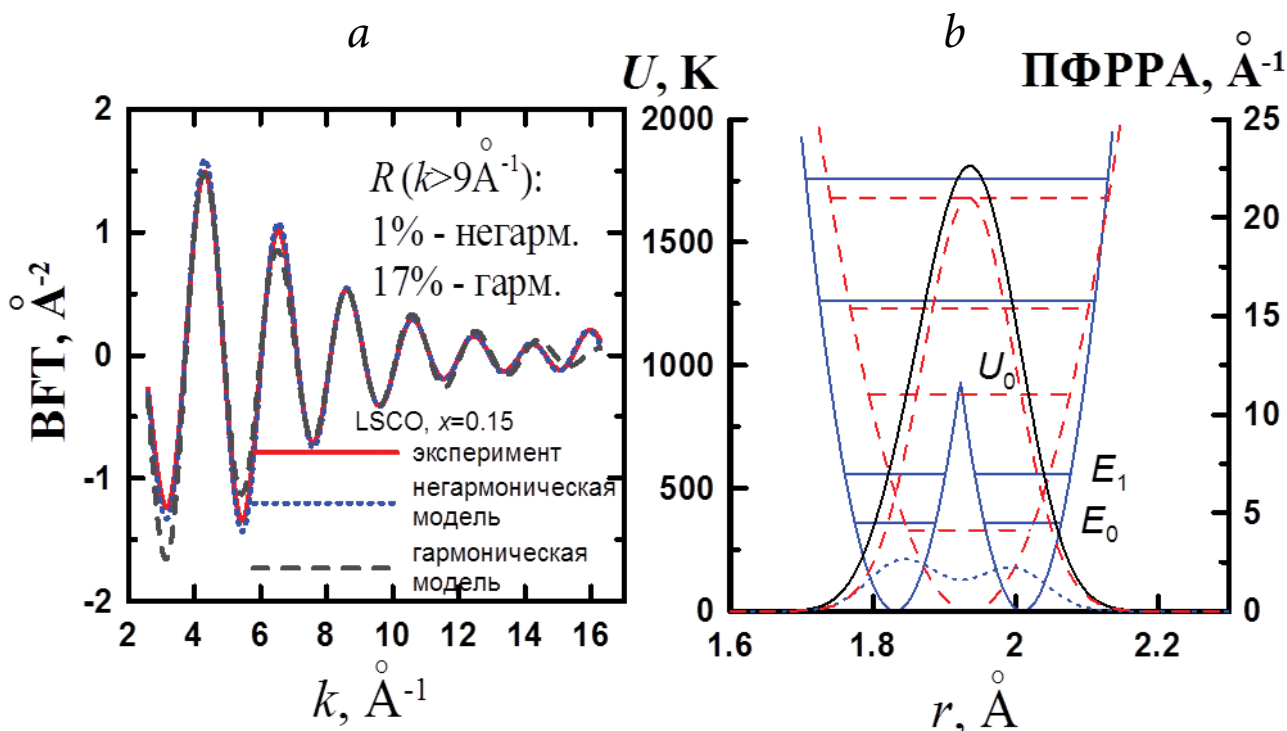
Рис. 3. а – Экспериментальная и модельные (негармоническая, с использованием двухъямного потенциала, и гармоническая) EXAFS-функции CuO-связи в сверхпроводящем La_{1.85}Sr_{0.15}CuO_4 (LSCO) – фурье-трансформанты (BFT) как функции волнового вектора k ; б – двухъямный и гармонический потенциалы с собственными энергетическими уровнями и ПФРРА как функции расстояния r . Разница нижних уровней E_1 - E_0 определяет частоту туннелирования в двухъямном потенциале.
