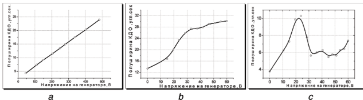
Рис. 3. Зависимость полуширины КДО от мощности ультразвука: а – кремний; б – фторид лития; в – парателлуриат.
