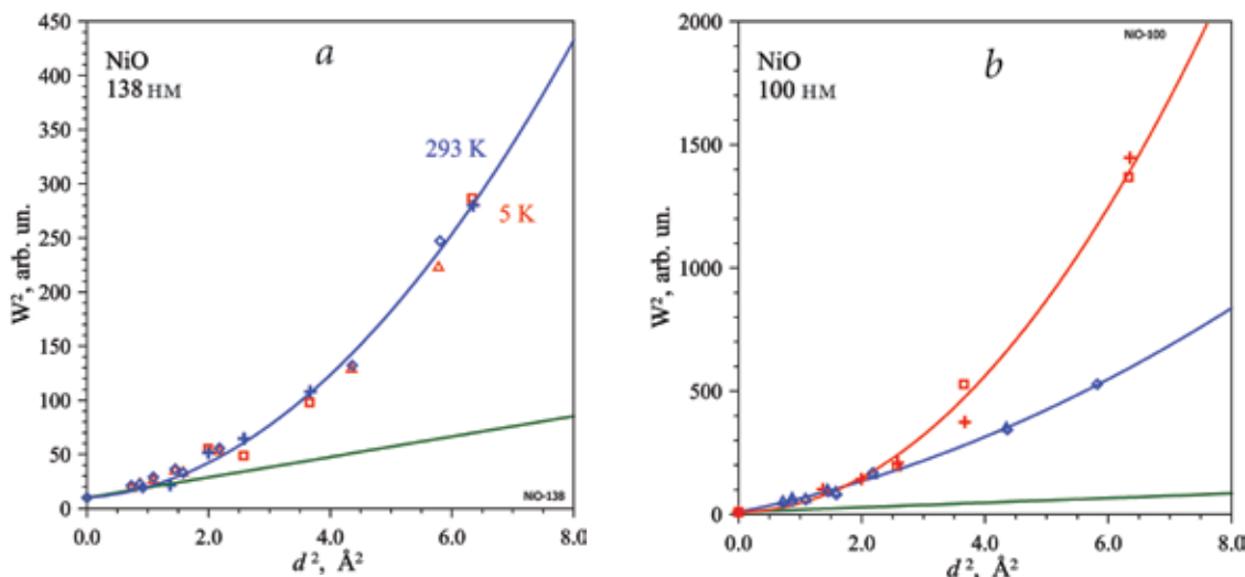
Рис. 5. Зависимости ширины ядерных (синие точки) и магнитных (красные точки) дифракционных пиков от межплоскостного расстояния для образцов NiO с размерами кристаллитов 138 (а) и 100 нм (b), измеренные при 293 и 5 К. Разрешению дифрактометра соответствует зеленая линия. Зависимости имеют параболический характер, указывающий на проявление эффекта размера. Для кристаллитов с L=138 нм ширины ядерных и магнитных пиков совпадают, тогда как для L=100 нм магнитные пики заметно шире ядерных.
