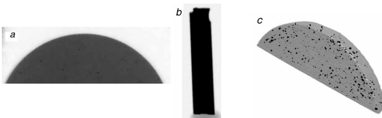
Рис. 2. Дефекты в сверхпроводниковых мишенях: интроскопия на монохроматическом нейтронном излучении \lambda=1.52 \text{ \AA} (установка АТОС) (а), фильтрованным синхротронном излучении (станция ЛИГА) (b) и трехмерная реконструкция образца по данным нейтронной томографии (с).
