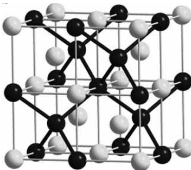
Рис. 1. Кристаллическая структура фазы высокого давления CeNi (подрешетки атомов церия и никеля показаны разными цветами).
