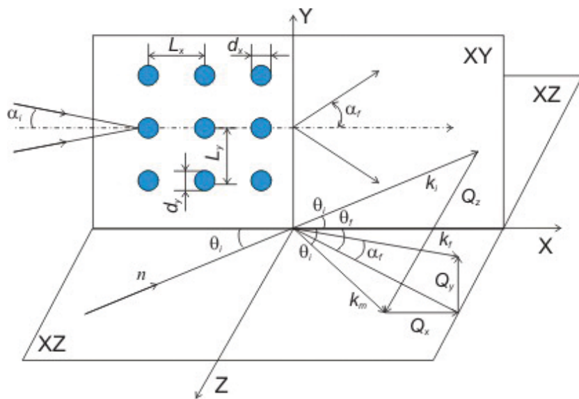
Рис. 1. Геометрия эксперимента по отражению и рассеянию поляризованных нейтронов от слоистой структуры, расположенной в плоскости XY.
