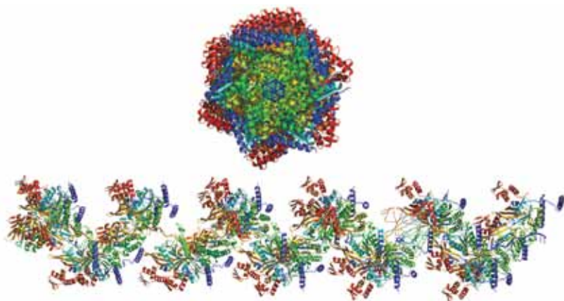
Рис. 2. Модель белка RecA из E. coli , состоящего из 33 мономеров, в комплексе с одДНК (здесь и далее одДНК – одонитевая ДНК) и АТФ. Цветом обозначена структура каждого мономера: красным – N-конец, синим – C-конец, промежуточные цвета – от N- до C-конца.
