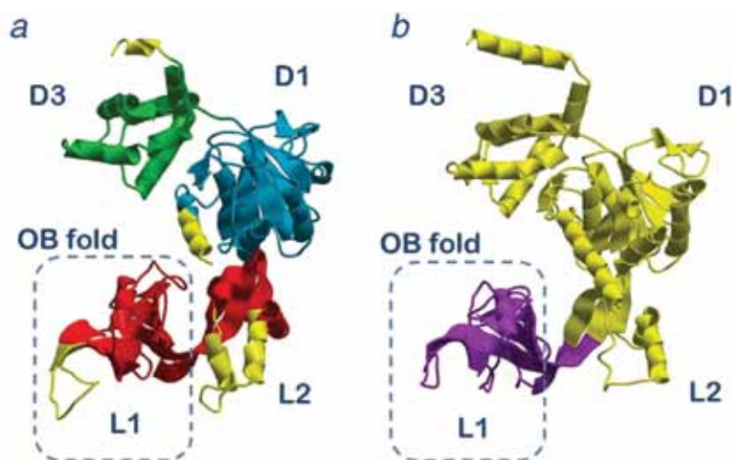
Рис. 7. Пространственные структуры мономерных форм белков TIR49a и TIR49b: а – кристаллическая структура TIR49a. Области D1, D2 и D3 показаны синим, красным и зеленым цветами соответственно. Неструктурированные петли L1 и L2 (обозначены желтым цветом) были реконструированы с использованием инструментов моделирования петель ICM-Pro; б – полноатомная пространственная структура TIR49a (построена на основе пространственной структуры гомологичного белка TIR49B).
