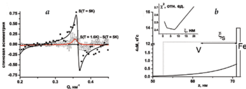
Рис. 3. а – Спиновая асимметрия (черный цвет) и разность спиновой асимметрии (красный цвет) для значений температуры 1.5 и 5.0 К: точки – эксперимент, линии – расчетные зависимости; б – магнитный профиль бислоя СП/ФМ при температуре ниже T_c .
