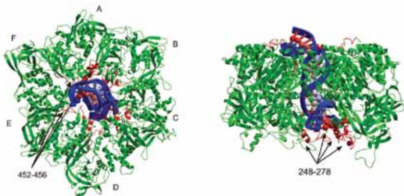
Рис. 9. Конечная конформация комплекса белка TIR49a с днДНК после 30 нс МД с разных ракурсов. Дополнительные по сравнению с начальной структурой элементы белка, находящиеся в прямом контакте с днДНК, показаны красным цветом.
