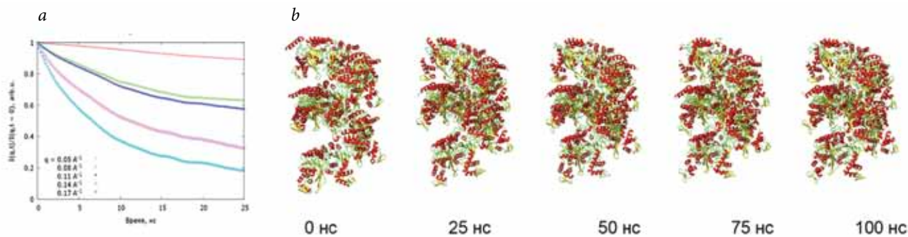
Рис. 5. Молекулярная динамика белка RecA: кривые релаксации сигнала НСЭ (а) и конформационные изменения в филаменте (b).
