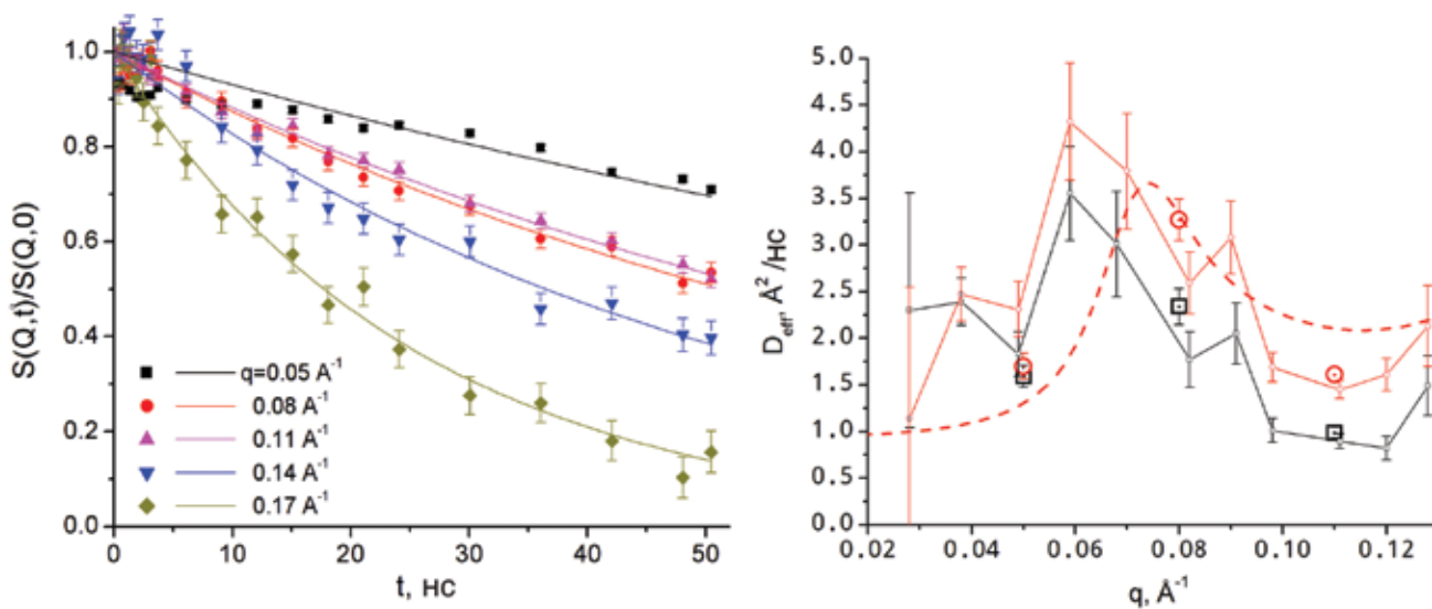
Рис. 6. Спектры НСЭ для филамента белка RecA. Данные JNSE (JCNS-MLZ, Мюнхен, Германия).
