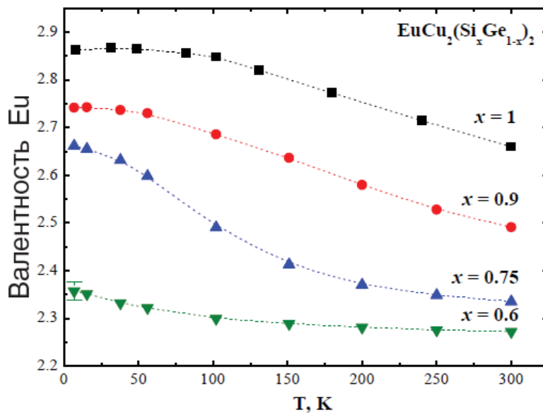
Рис. 4. Температурные зависимости валентного состояния европия для разного содержания германия в EuCu_2(SixGe_{1-x})_2 .
