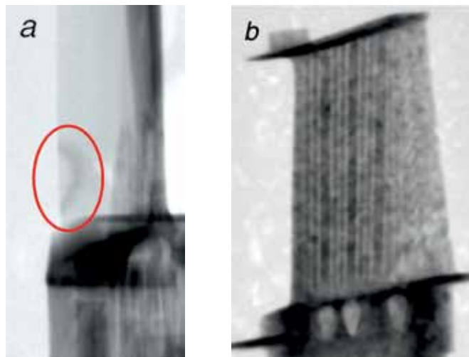
Рис. 5. Дефекты внутреннего строения различных типов турбинных лопаток: включение фазы иной ориентации (выделено красным) (а) и неоднородности в каналах (б).
