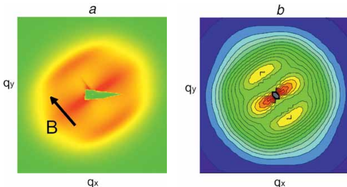
Рис. 3. Сравнение экспериментальной (a) и расчетной (b) анизотропных двумерных картин малоуглового рассеяния СИ для магнитной жидкости на основе наночастиц кобальта в толуоле, помещенной во внешнее магнитное поле B=160 мТл; направление поля показано на рисунке 2a.
